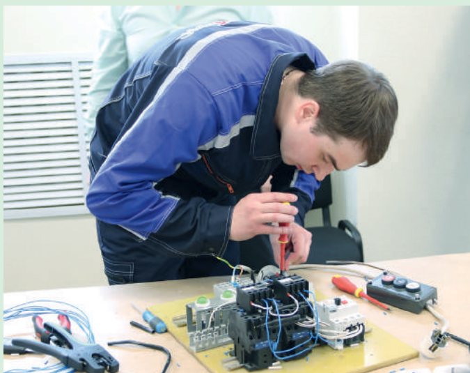
Конкурсант Виталий Плехов выполняет практическое задание № 2, собирая схему реверсивного пускателя
